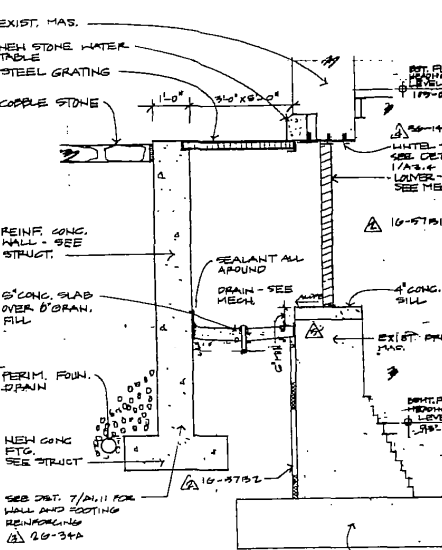
SECTION THRU AREAWAY (1) A1.7 SCALE: 1/2" = 1'-0"
