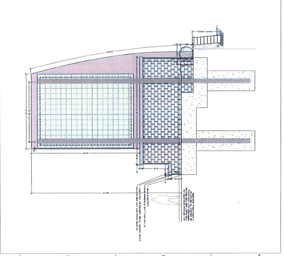
7 MONUMENT SIGN SCALE: 1/8" = 1'-0" SECTION
